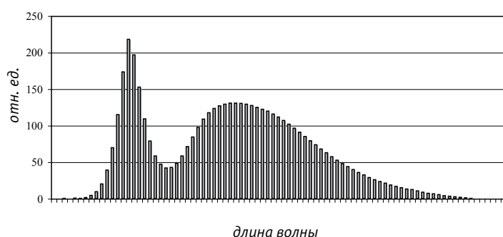
Спектр лампы LEDLAMP T8
